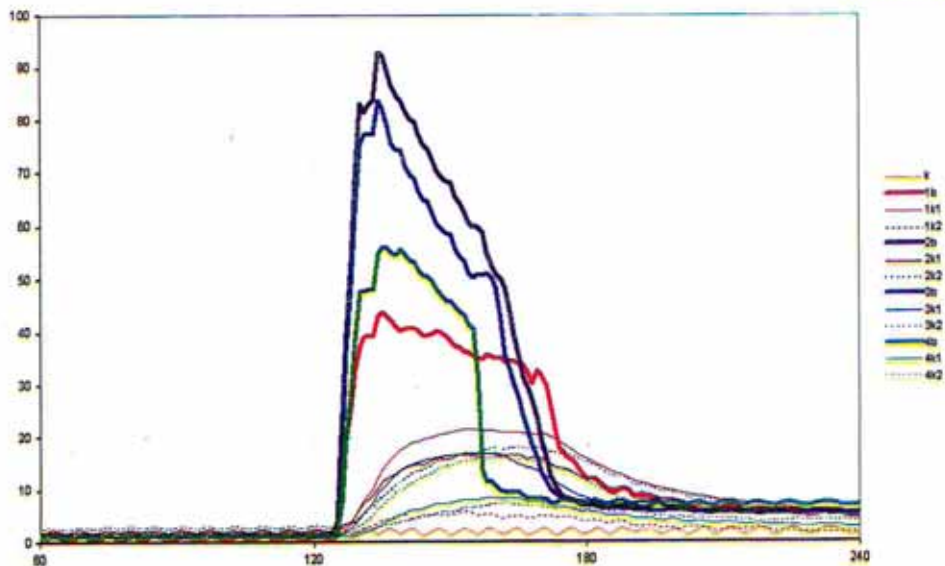
A hőmérséklet alakulása a kürtőben "tűzteszt" vizsgálatok, a tűzgátló berendezés működésekor.
